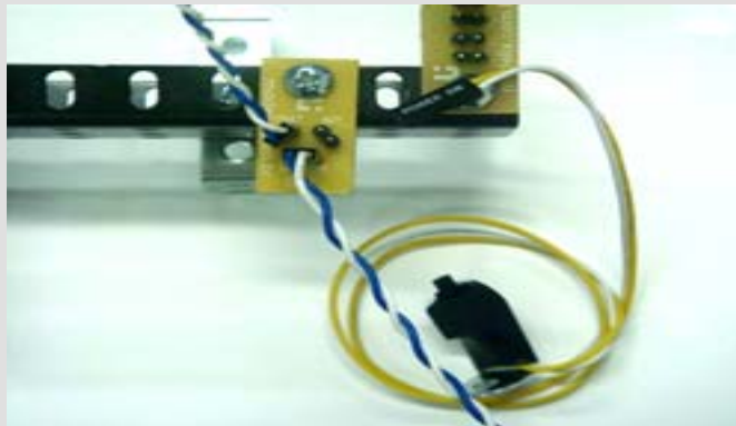
Figura 1: Desconecte o interruptor do INT do RELE, para fazer a adaptação.
